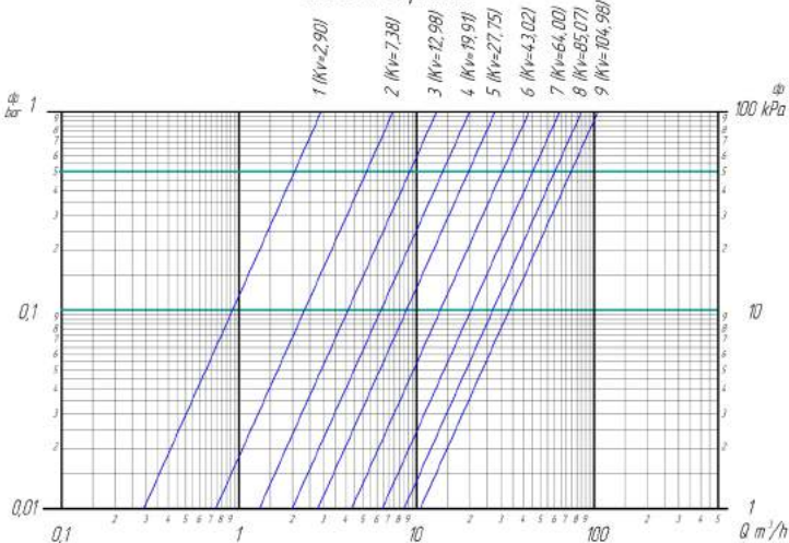
DN125 W-образный
