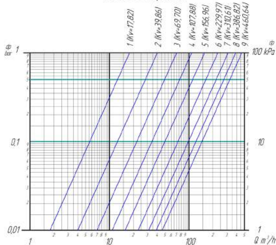
DN150 W-образный
