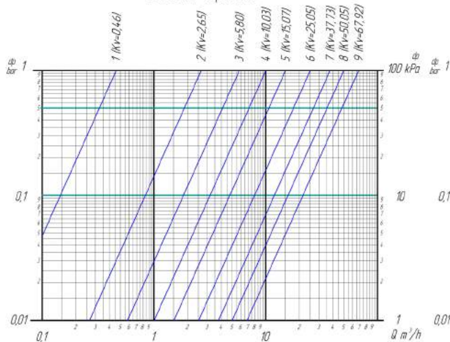
DN100 W-образный
