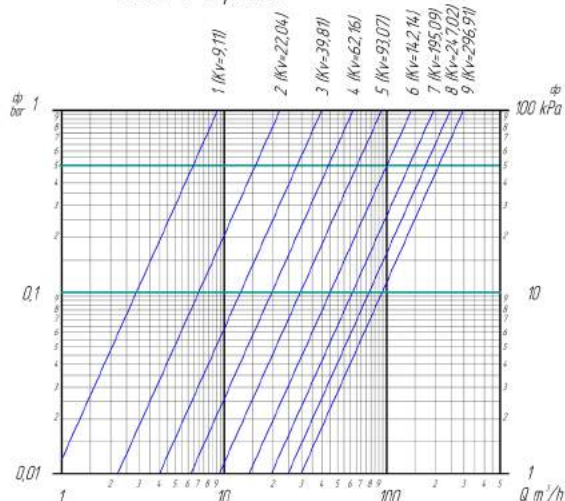
DN125 W-образный
